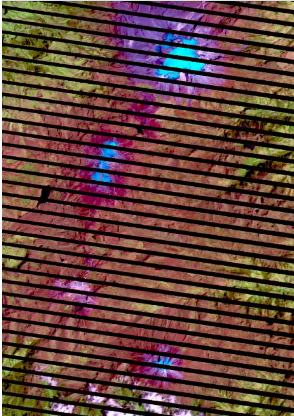
Landsat Febrero de 2004, C542
