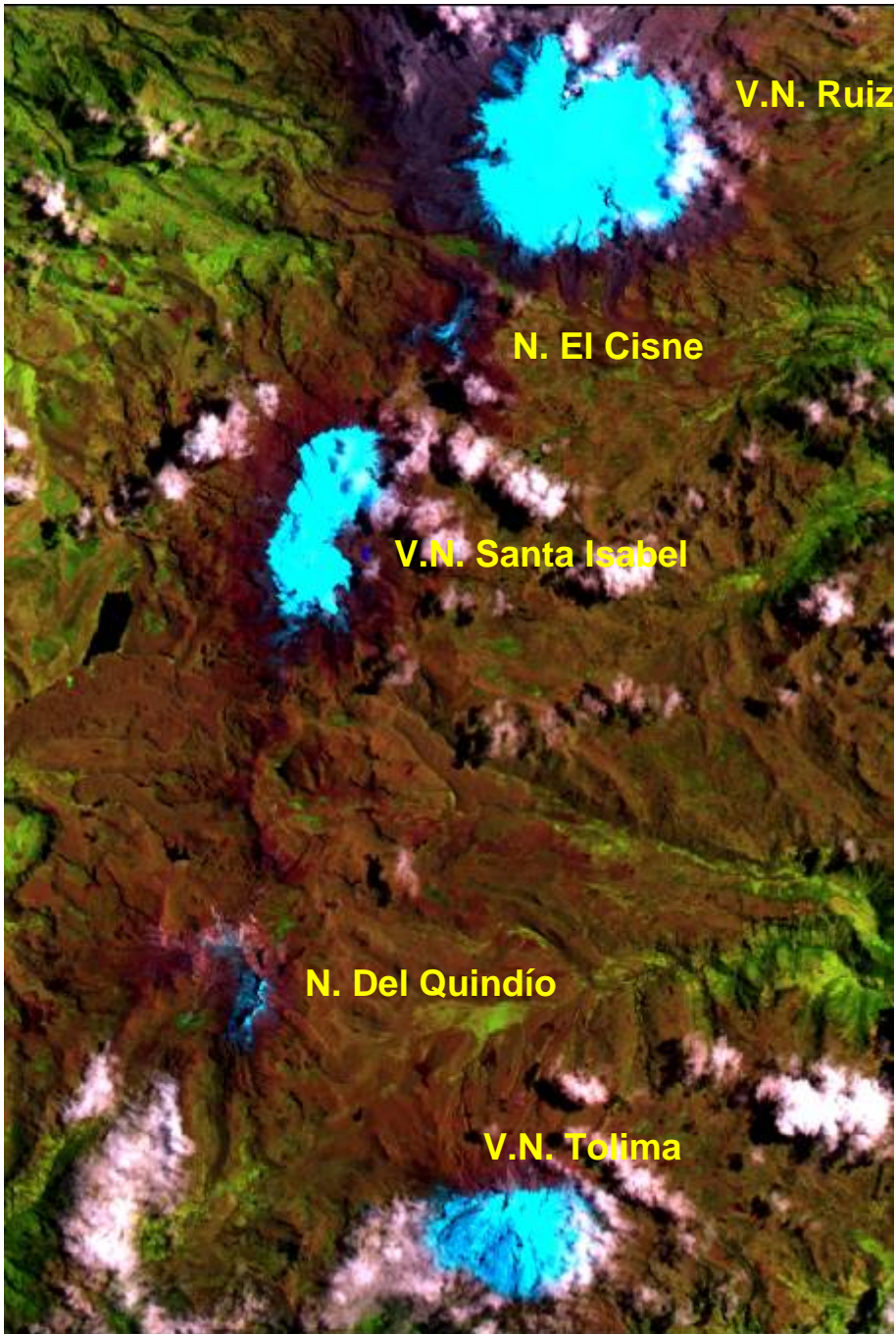
Landsat Agosto de1989, C542
