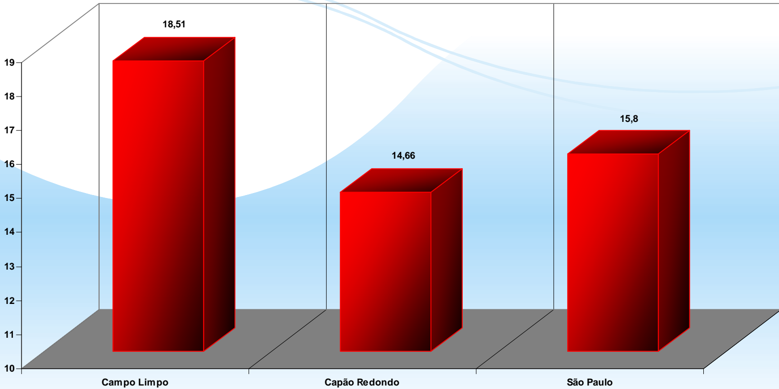
Taxa de Mortalidade Infantil - 2008
